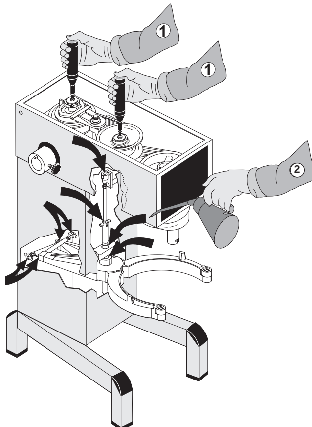
fig.5 Smøring af trinkløst gear og øvrige bevægelige dele
