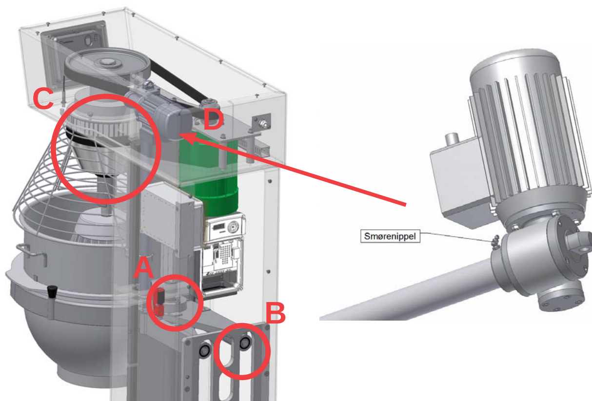
Fig. 1 Smøreoversigt
