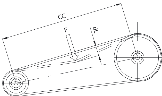
Fig. 2. Remtilspænding.
