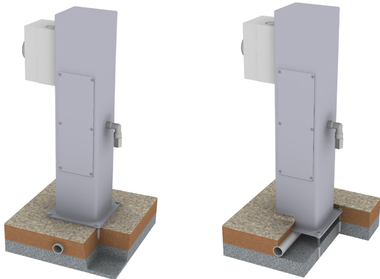
Søjle placeret på færdigt gulv.
